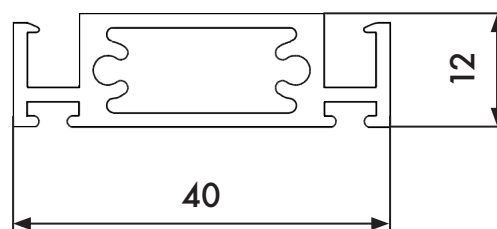
Traverse de renfort
