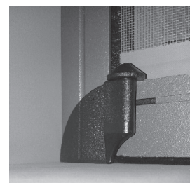
Pieds de coulisse réglables
