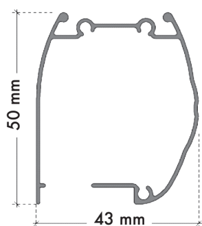
Coupe du boîtier
