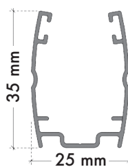
Coupe de la coulisse
