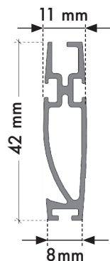
Coupe de la barre de charge
