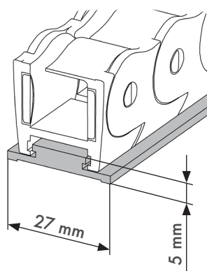
Coupe du guide bas
