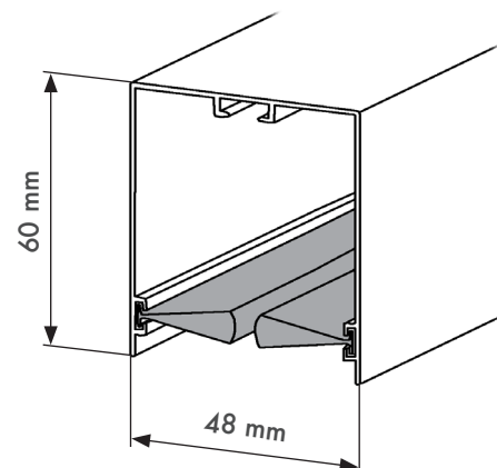
Coupe du rail haut
