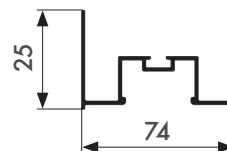
Coupe du profil
